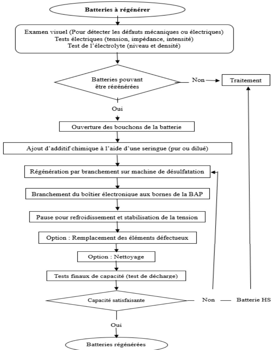
Figure 3 : Synoptique type du procédé Combiné [10]
