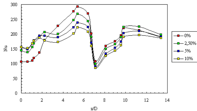
Figure 15 : L'évolution du nombre de Nusselt en fonction de l'abscisse Z/D à densité de flux de chaleur ( 9480 \text{ W/m}^2 ) et à nombre de Reynolds généralisé ( R_g = 1028 ) constants
