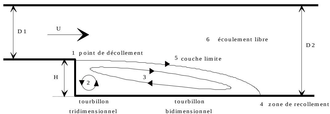
Figure 4 : Écoulement turbulent d'eau en aval d'une marche descendante (Cf. Fagla et al., 2013) [10]
