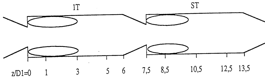
Figure 8: Zone de recirculation pour 550 \leq \text{Reg} \leq 900 dans la géométrie complexe de la veine d'essais
