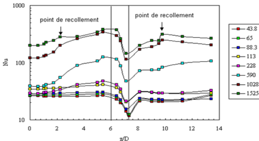
Figure 9 : Evolution du nombre de Nusselt à densité de flux constante soit 5024 \text{ W/m}^2 pour différentes valeurs du nombre de Reynolds généralisé \text{Reg}
