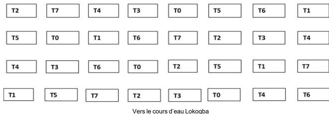
Figure 2 : Dispositif expérimental de l'essai Experimental design of the test
