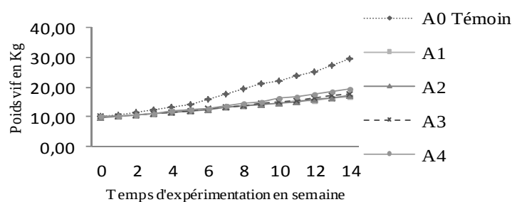
Figure 2 : Evolution du poids pondéral en fonctions des traitements alimentaires.
