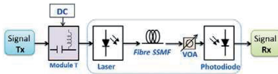
Figure 4.1 : Schéma de base de la liaison IM/DD simulée.
