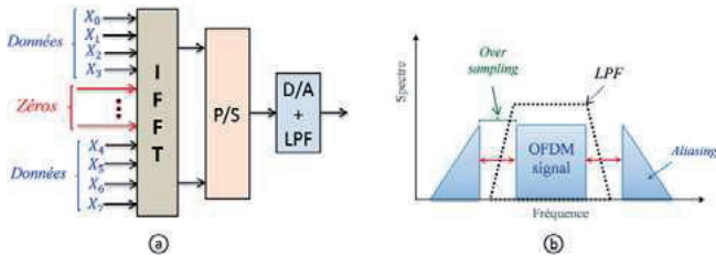
Figure 2.21 : (a) Implémentation de l'Over-sampling sur IFFT, (b) Effet sur le spectre.
