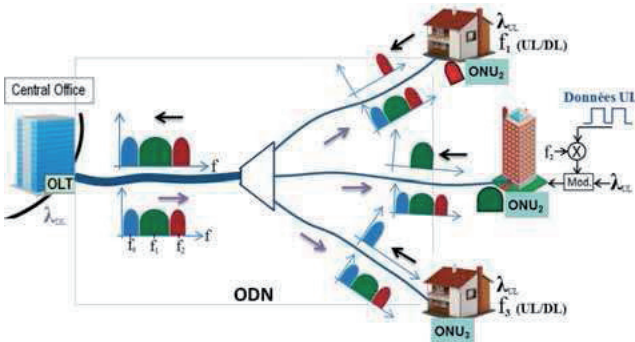
Figure 1.6: Exemple d'une technologie FDM/FDMA.
