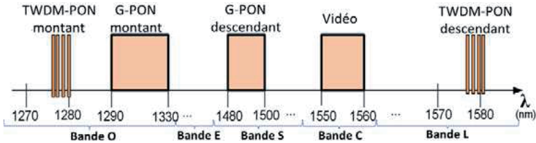
Figure 1.12: Réutilisation des longueurs d'onde du XG-PON en TWDM [12].
