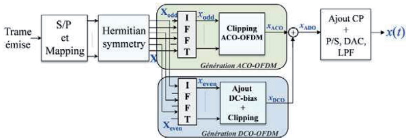
Figure 3.24 : Schéma de principe d'un émetteur ADO-OFDM.
