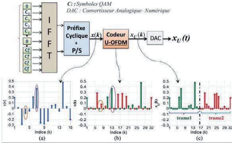
Figure 3.14 : Schéma de principe d'un émetteur U-OFDM.
