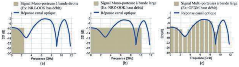
Figure 2.15 : Spectre électrique d'un signal : (a) Mono-porteuse bas débit, (b) Mono-porteuse haut débit, (c) Multi-porteuses haut débit.
