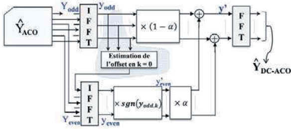
Figure 3.19 : Schéma de principe d'un démodulateur DC-ACO.
