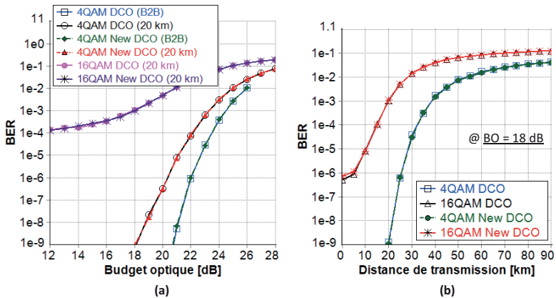
Figure 4.22 : Comparaison DCO vs New DCO pour différentes QAM : (a) BER vs BO en B2B et 20 km, (b) BER vs distance de transmission pour BO = 18 dB à débits identiques.
