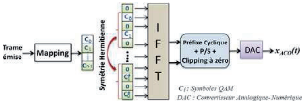
Figure 3.8 : Schéma de principe d'un émetteur ACO-OFDM.
