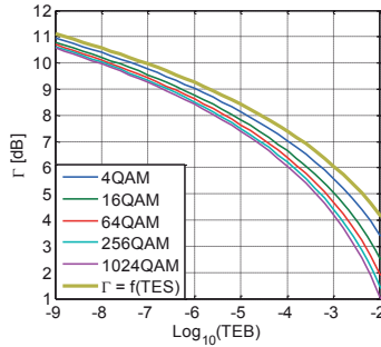
Figure 2.26 : \Gamma en fonction du BER et comparaison avec la référence \Gamma = f(\text{SER}) .
