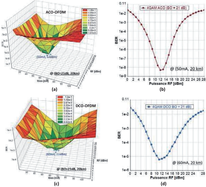
Figure 4.15 : Performances obtenues à 20 km pour BO = 21 dB : (a) BER fonction de la puissance RF (signal ACO) et de I_{bias} , (b) BER fonction de la puissance RF (signal ACO) pour I_{bias} = 50 \text{ mA} , (c) BER vs puissance RF (signal DCO) et de I_{bias} (d) BER vs puissance RF (signal DCO) pour I_{bias} = 60 \text{ mA} .
