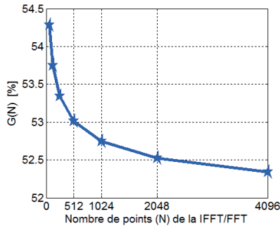
Figure 3.32 : Courbe G(N) fonction de N .
