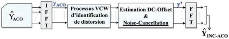
Figure 3.27 : Schéma de principe d'un démodulateur INC-ACO.
