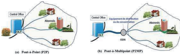
Figure 1.3: Méthodes d'acheminement des données dans les PON.
