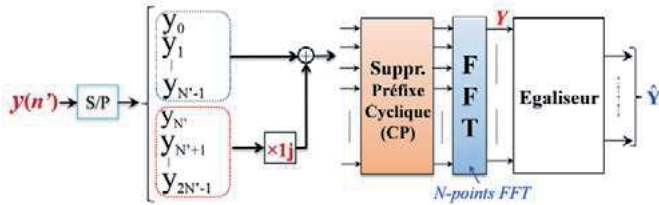
Figure 3.30 : Schéma de principe d'un démodulateur New OFDM.
