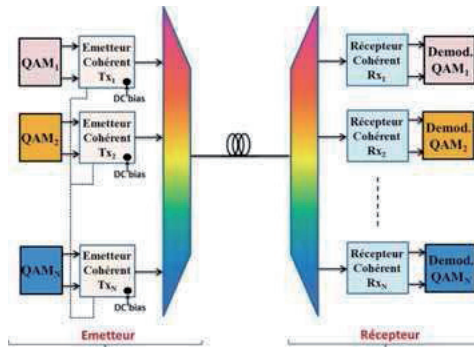
Figure 3.3 : Schéma de principe d'une liaison OFDM tout-optique.
