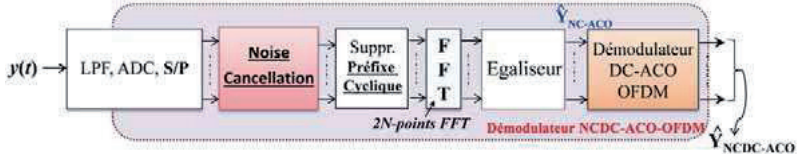
Figure 3.22 : Schéma de principe d'un démodulateur NCDC-ACO.
