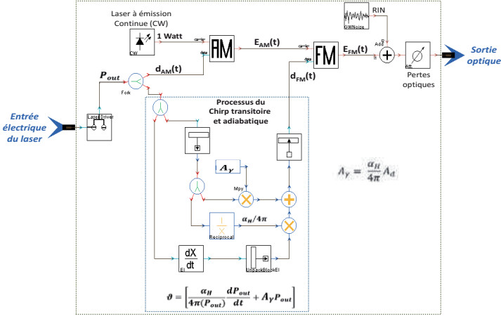
Figure 4.3 : Modèle phénoménologique du laser DFB avec VPI.
