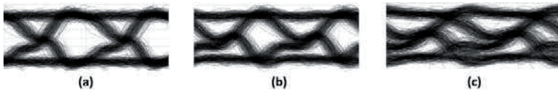
Figure 4.11: Diagrammes de l'œil obtenus pour 20 km et un débit de : (a) 5 Gb/s, (b) 7,5 Gb/s, (c) 10 Gb/s.
