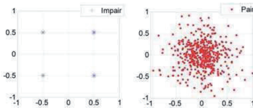
Figure 3.11 : Constellation reçue en sortie d'un canal plat « sans bruit AWGN ».
