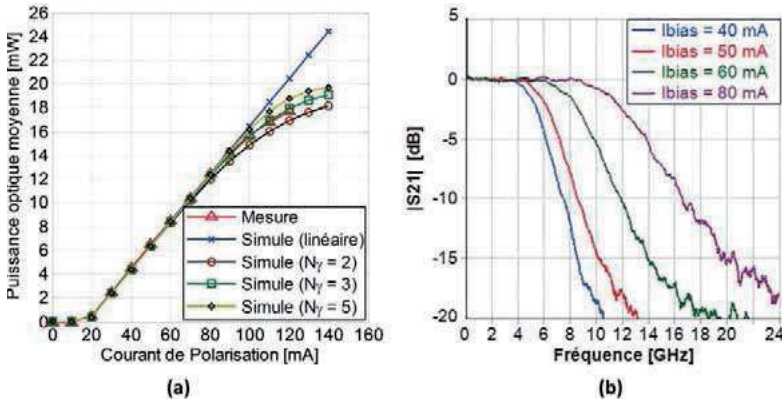
Figure 4.4 : (a) Caractéristiques P=f(I) du laser DFB étudié - (b) réponse fréquentielle en fonction du courant de polarisation ( I_{bias} ).
