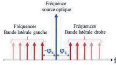
Figure 2.2 : Spectre optique d'un signal modulé IM.
