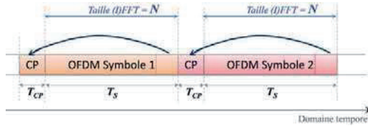
Figure 2.22 : Implémentation du préfixe cyclique en OFDM.
