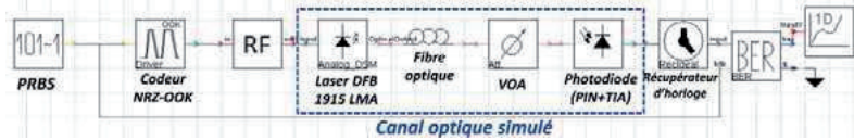
Figure 4.9: Schéma de simulation d'une liaison NRZ-OOK.
