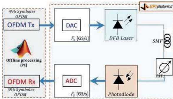
Figure 4.12 : Liaison OFDM sur fibre optique.
