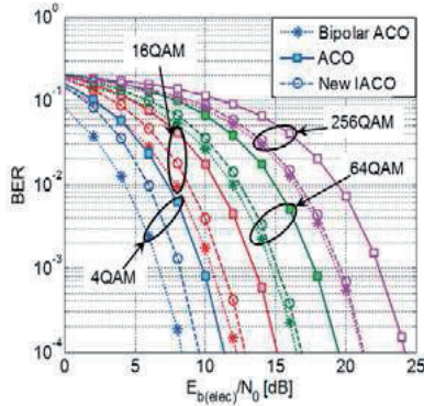
Figure 3.36 : Performances des techniques New IACO, ACO-bipolaire et ACO en fonction de E_{b(elec)}/N_0 .
