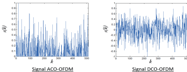
Figure 4.14 : Signal ACO-OFDM et DCO-OFDM générés avec MATLAB.
