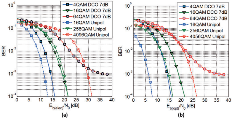
Figure 3.16 : Performances des techniques U-OFDM et DCO-OFDM dans un canal plat AWGN pour différentes QAM : (a) en fonction de E_{b(elec)}/N_0 , (b) en fonction de E_{b(opt)}/N_0 .
