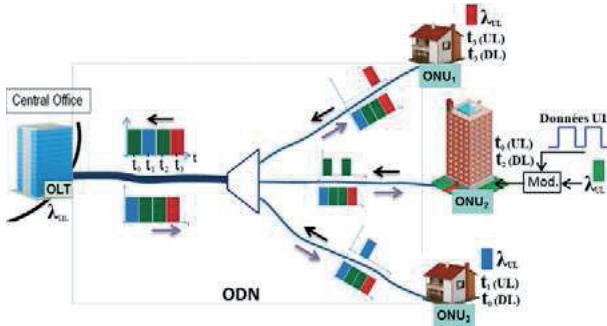
Figure 1.5: Exemple d'une technologie TDM/TDMA.
