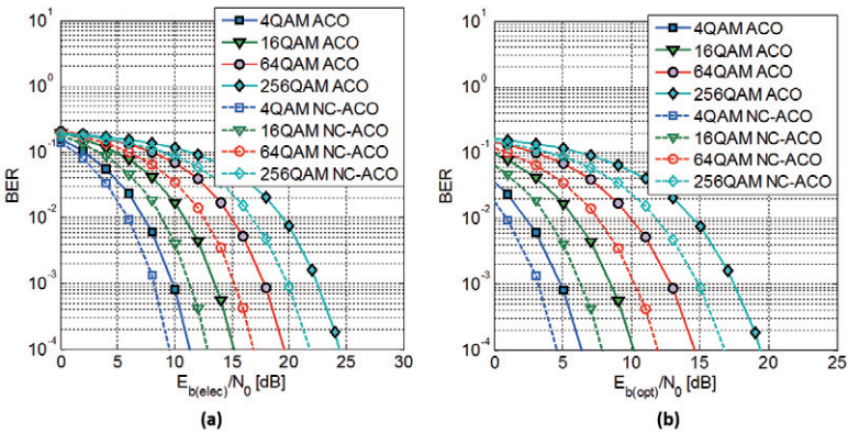
Figure 3.18 : Performances des techniques NC-ACO et ACO-OFDM dans un canal plat AWGN pour différentes QAM: (a) en fonction de E_{b(elec)}/N_0 , (b) en fonction de E_{b(opt)}/N_0 .
