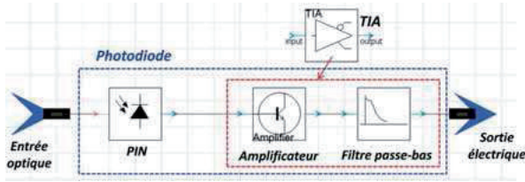
Figure 4.5 : Modèle VPI du récepteur optique (PIN+TIA).
