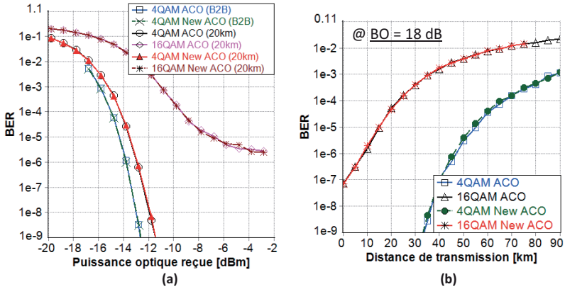
Figure 4.23 : Comparaison ACO vs New ACO pour différentes QAM : (a) BER vs POR en B2B et 20 km, (b) BER vs distance de transmission pour BO = 18 dB à débits identiques.
