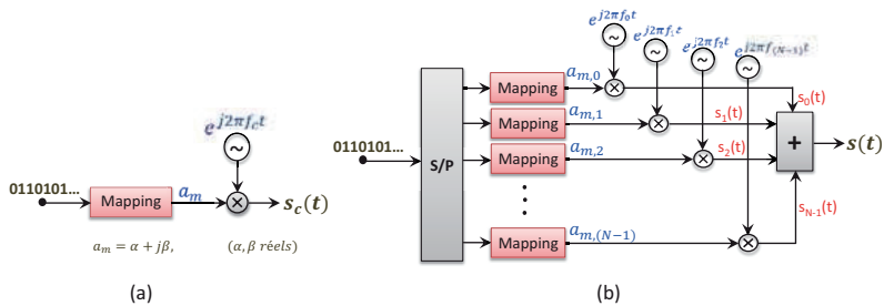
Figure 2.16 : Comparaison entre techniques de modulation - (a) Mono-porteuse, (b) Multi-porteuses (exemple du FDM).
