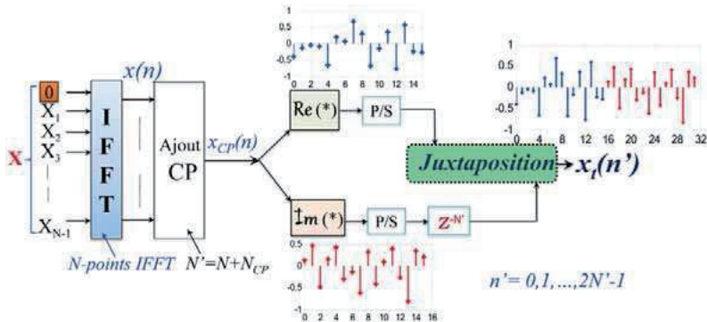
Figure 3.29 : Schéma de principe d'un modulateur New OFDM.
