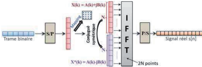
Figure 2.25 : Principe de fonctionnement de la symétrie hermitienne.
