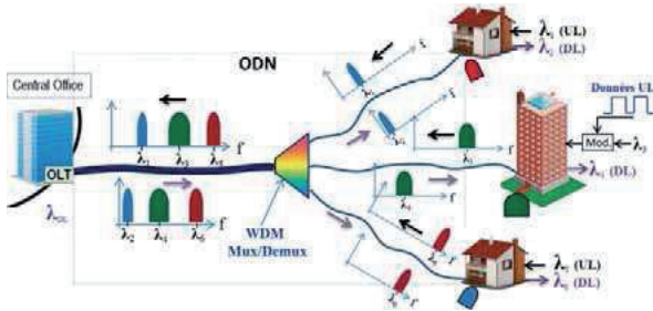
Figure 1.7: Exemple de technologie WDM/WDMA.
