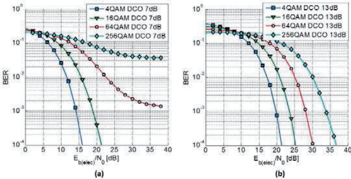
Figure 3.6 : Performances BER vs E_{b(elec)}/N_0 obtenues avec la technique DCO pour un canal plat AWGN lorsque : (a) DC_{Bias}(dB) = 7\text{ dB} , (b) DC_{Bias}(dB) = 13\text{ dB} .
