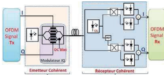
Figure 3.2: Schéma de principe d'une liaison OFDM cohérent.
