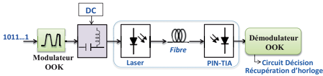
Figure 2.10 : Schéma d'une liaison IM/DD à modulation NRZ-OOK.
