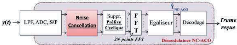
Figure 3.17 : Schéma de principe d'un démodulateur NC-ACO.
