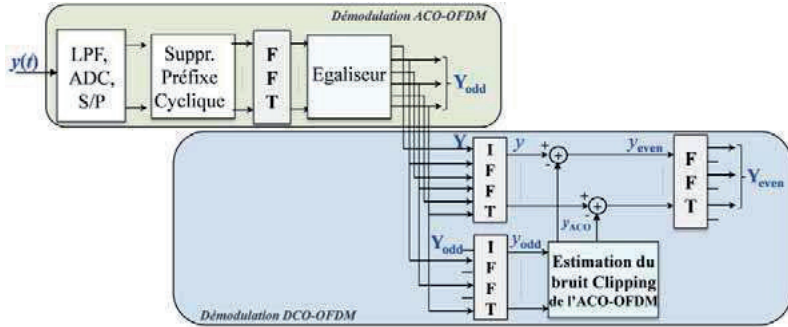
Figure 3.25 : Schéma de principe d'un récepteur ADO-OFDM.
