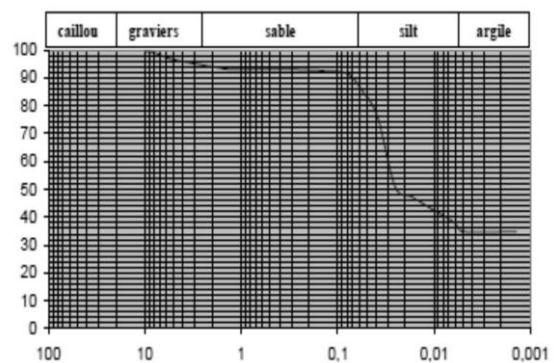
Figure 3 : Courbe granulométrique de l'argile de Zogbodoméy
