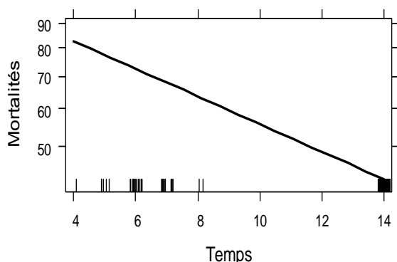
Temps effect plot
