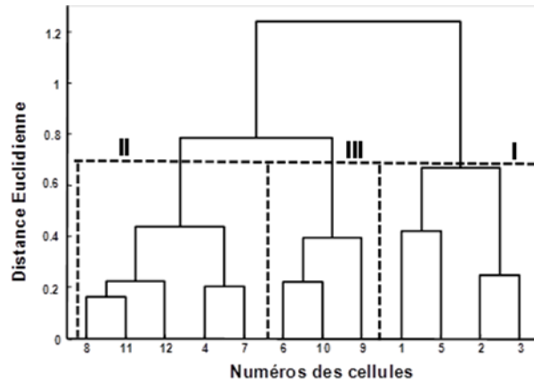
Figure 2 : Classification hiérarchique des cellules de la SOM avec la méthode de Ward
