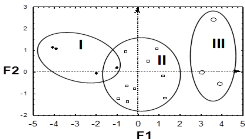
Figure 5 : Analyse factorielle discriminante portant sur les groupes (I à III)
