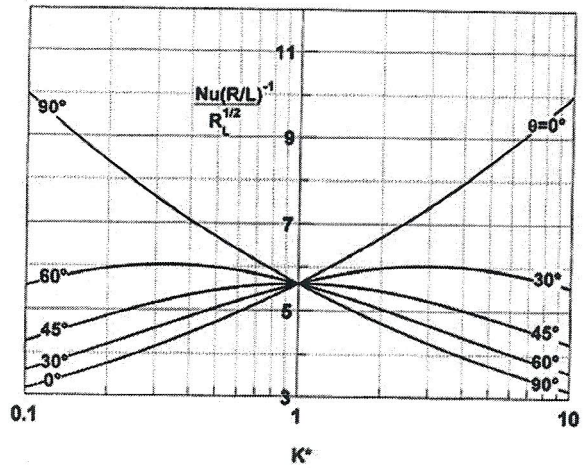
Figure 6. Effets du rapport d'anisotropie K^* et de l'angle d'orientation des axes principaux sur le nusselt Nu .
