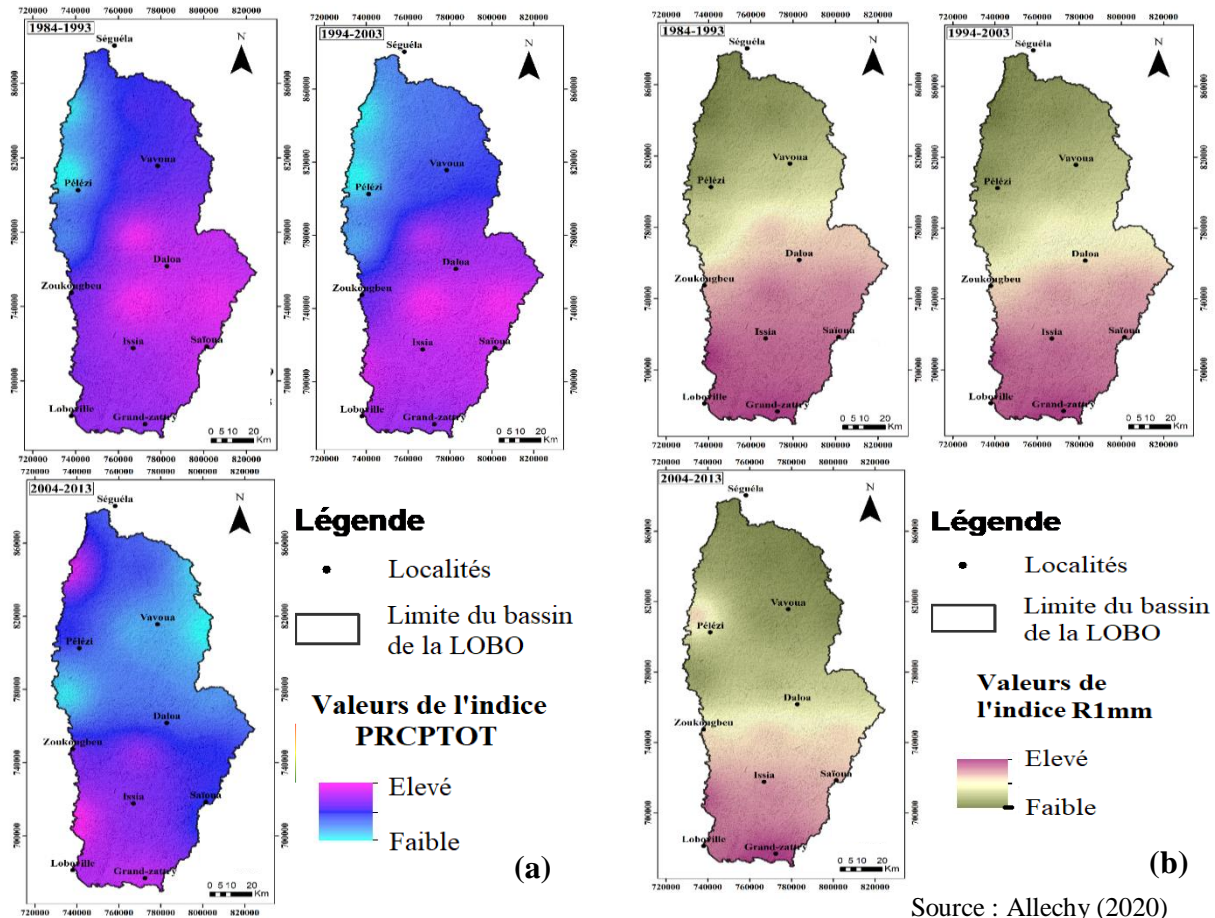
Fig.2 : Evolution spatio-temporelle du cumul annuel de précipitations (a) et du nombre de jours pluvieux (b) dans le bassin de la Lobo de 1984 à 2013
