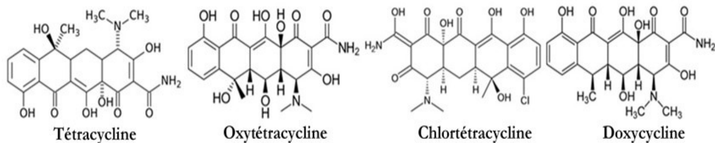
Figure 1b : Structure chimique des tétracyclines
