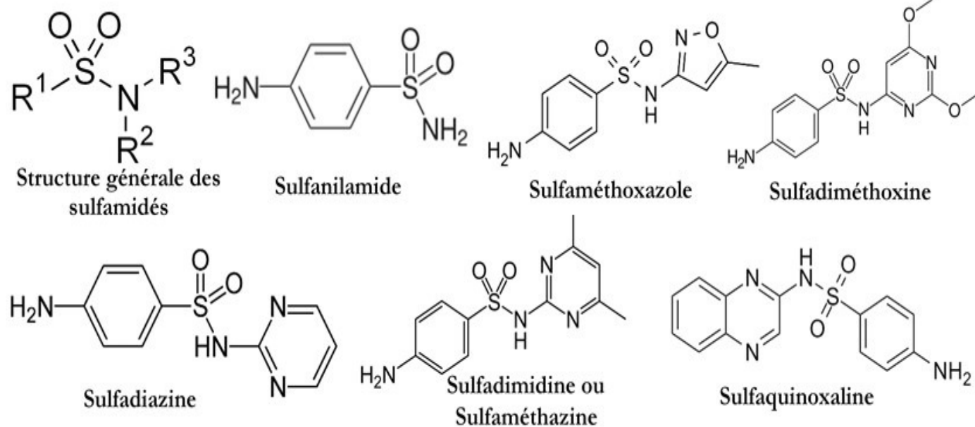
Figure 1a : Structure chimique des sulfamidés
